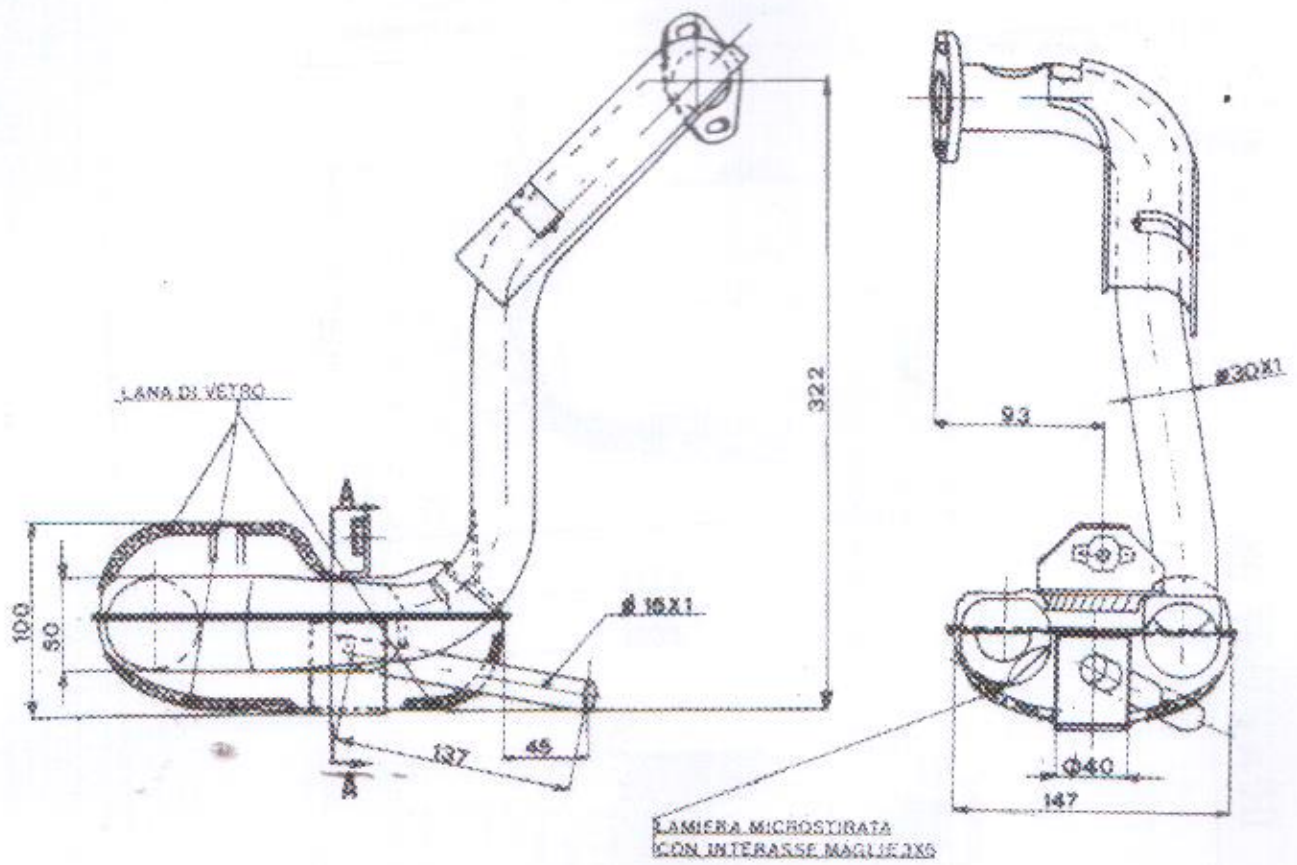
SEZ. A-A
